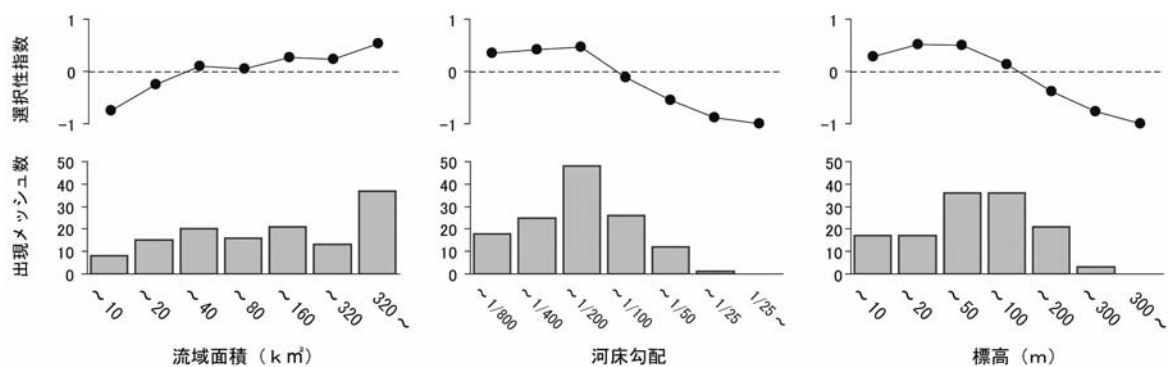
流域面積，河床勾配，標高別にみた出現メッシュ数，および選択性指数
